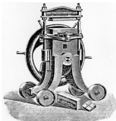
Figur 12. Svinghulsefterpresse fra firmaet Badischer Maschinenfabrik (Bock 1901)
