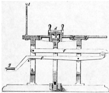
Figur 9. Simpel efterpresse af jern. Via vægtstangsarmen overføres arbejderens vægt fra pedalen til stemplet i bunden af formen. (von Waldegg, 1891)
